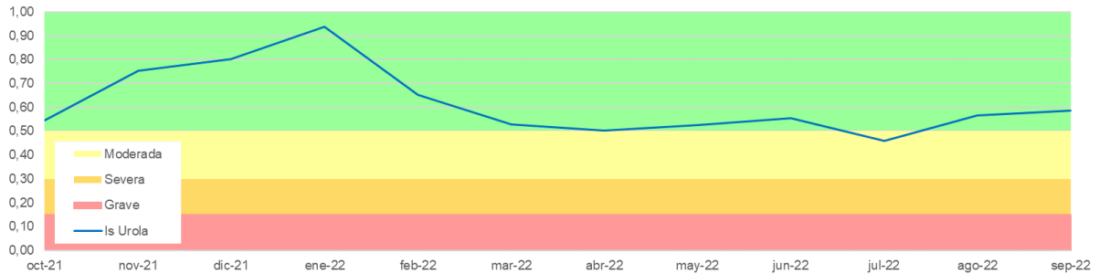
Figura nº17 Evolución del indicador de sequía. UT 08 Urola
