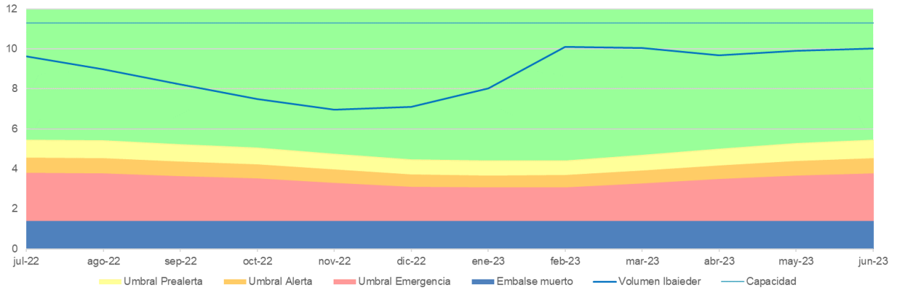
Figura nº21 Evolución del volumen (hm 3 ). Embalse de Ibaieder
