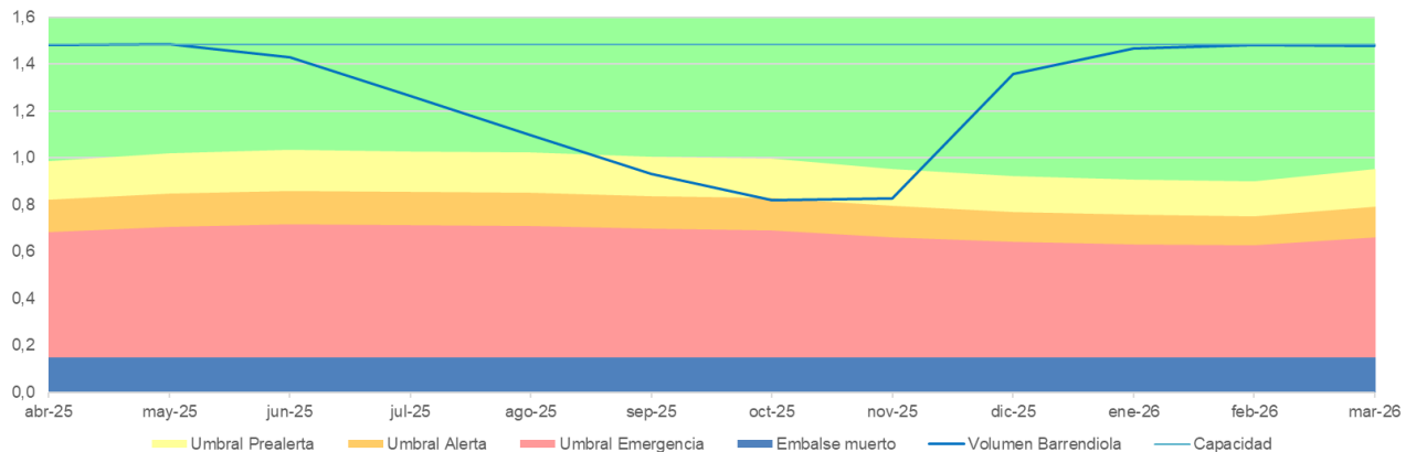
Figura nº20 Evolución del volumen (hm³). Embalse de Barrendiola
